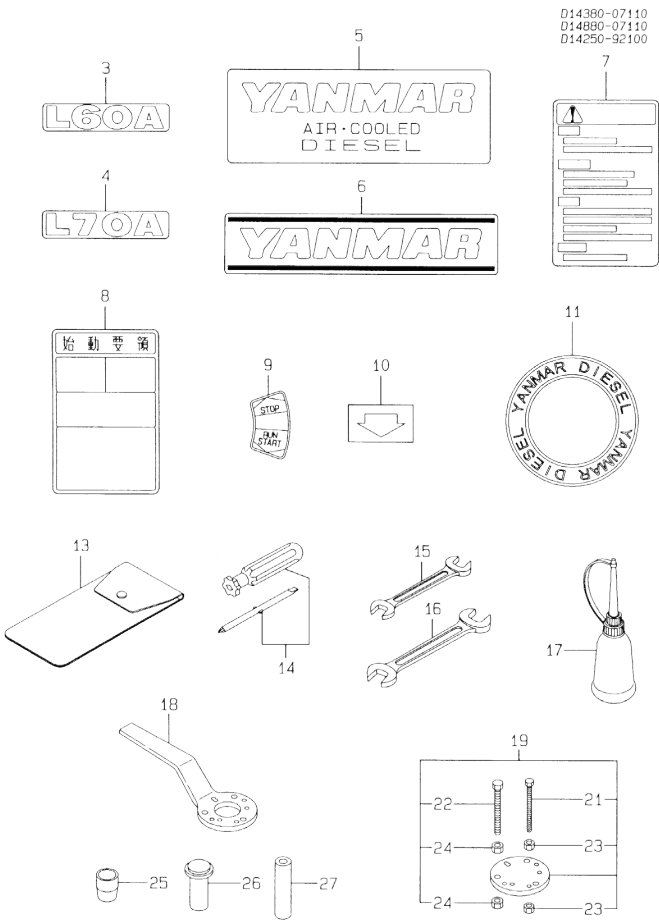
Fig.10. TOOL & LABEL
